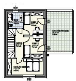
Obergeschoss 45,66 m²
