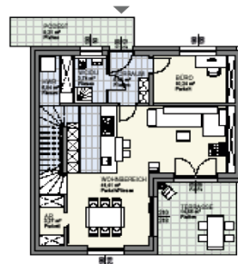
Erdgeschoss 73,52 m²
